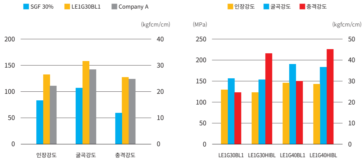
기계적 물성 비교
